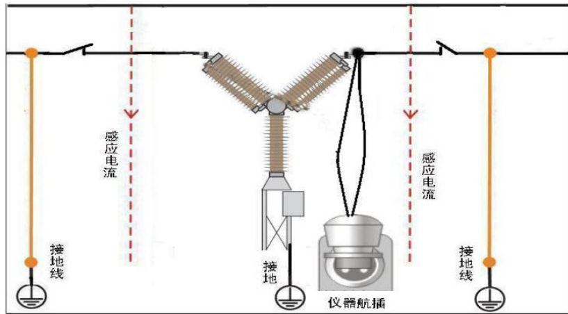
双端接地示意图
